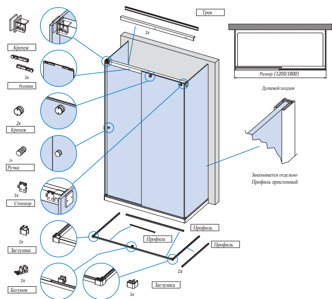
VX-1000 тип 3 Душевая кабина П-образная
