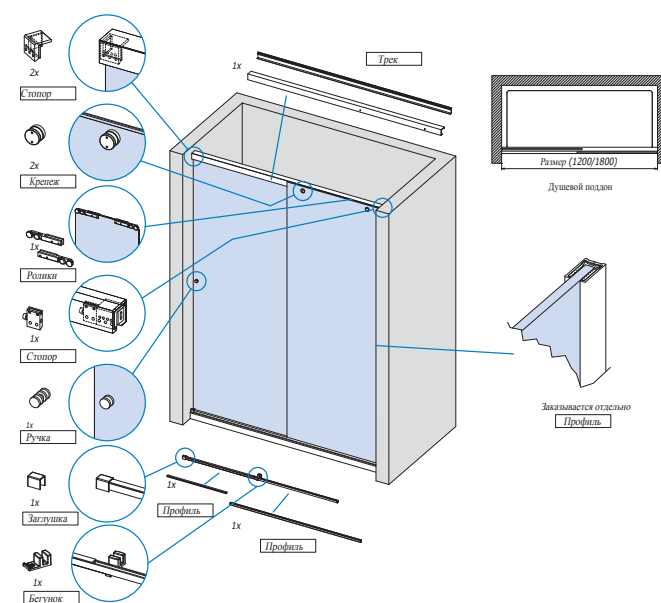
VX-1000 тип 4 Душевая кабина с двумя стационарными стеклами
