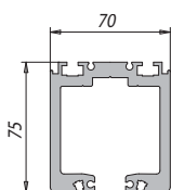
Несущий трек
