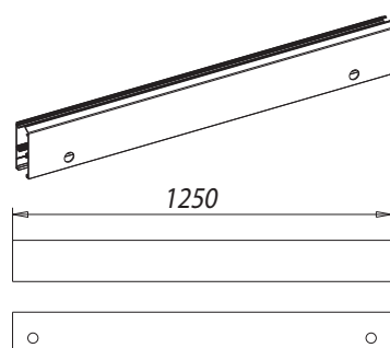
Накрывающая планка
